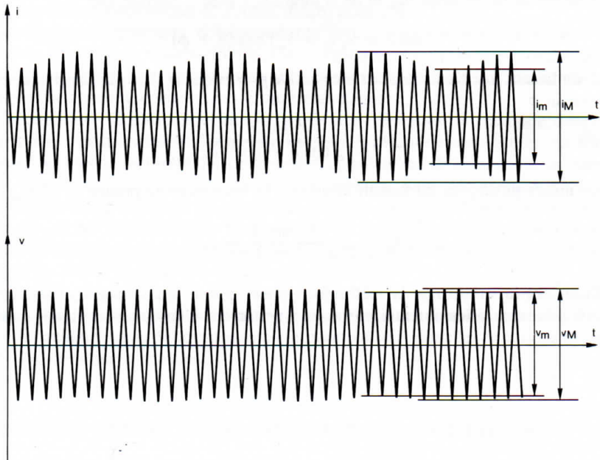
Fig. 6.5. — Oscillogramme de l'essai à faible glissement, pour la mesure de x_d et x_q .
