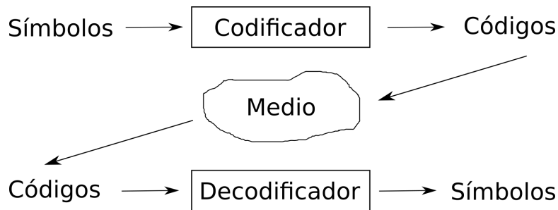
Figura 1: Esquema general de trabajo, un mensaje compuesto por N símbolos es codificado por el Codificador , generando k códigos que son transmitidos a través de un canal o almacenados en memoria. En el esquema estos dos casos están representados por la nube llamada Medio . El Decodificador convierte los códigos recibidos a través del canal de comunicación o leídos de memoria y los convierte nuevamente en símbolos que pueden ser interpretados por un humano.
