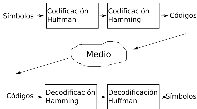
Figura 2: Esquema final donde se pueden probar las dos codificaciones implementadas en el curso, la de Huffman para comprimir y la de Hamming para detectar y corregir errores. Los códigos son transmitidos a través de un canal o almacenados en memoria. En el esquema estos dos casos están representados por la nube llamada Medio .
