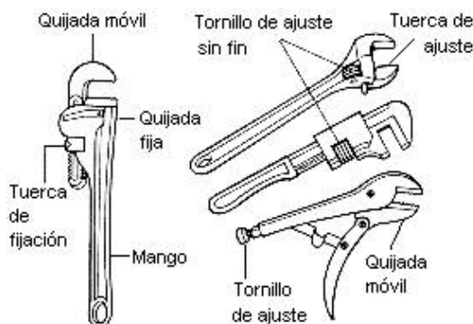
Fig. 4: Llaves de boca ajustable y sus partes
