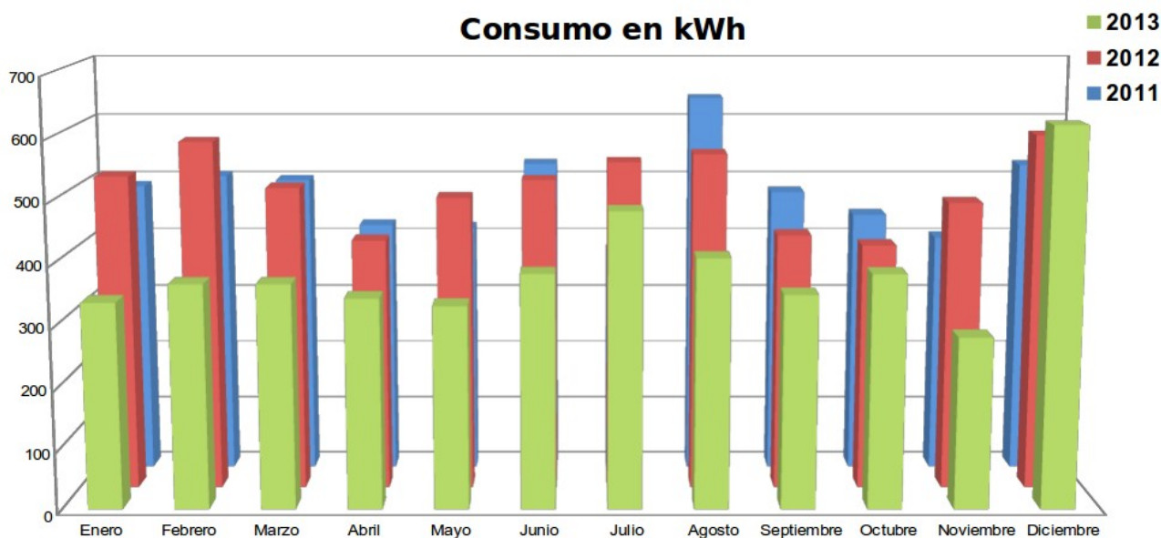
Fig. 2 – Consumo mensual del hogar. 2011 y 2012 sin sistema solar. 2013 con sistema solar.
