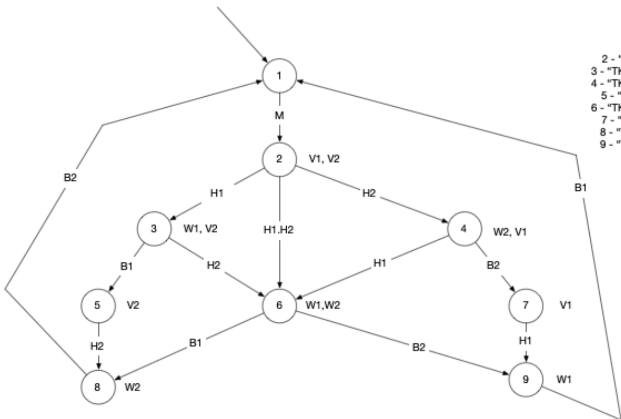
Grafcet (SFC)
