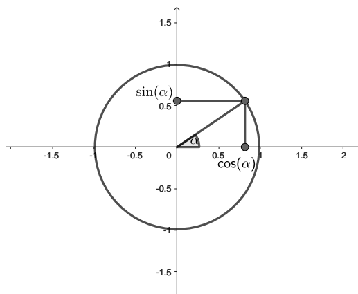
Figura 1: Círculo trigonométrico.
