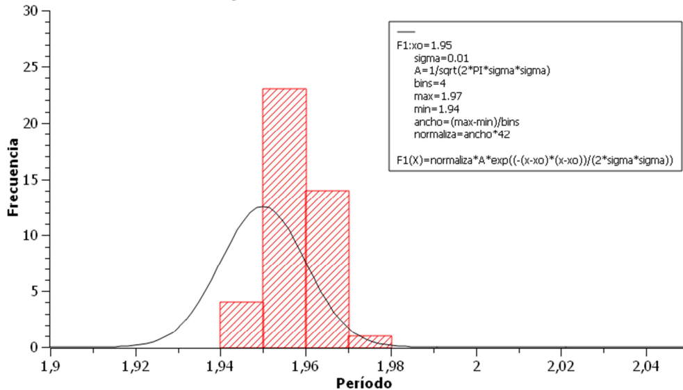
Histograma del período medido con el cronómetro (con datos descartados) y curva Gaussiana normalizada
