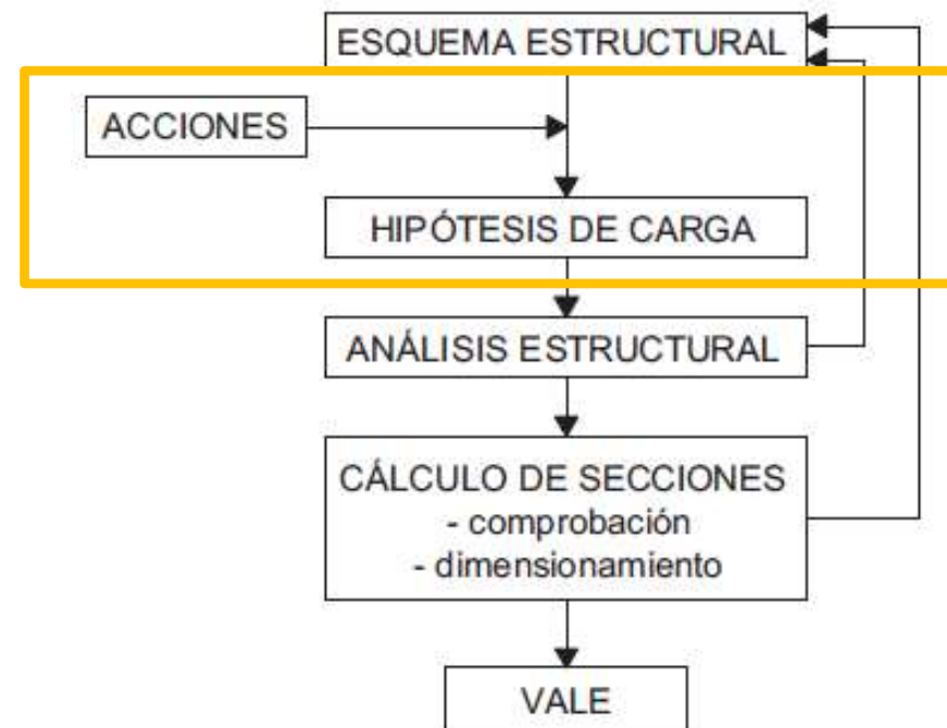
Figura 13.1 Proceso de cálculo de una estructura
