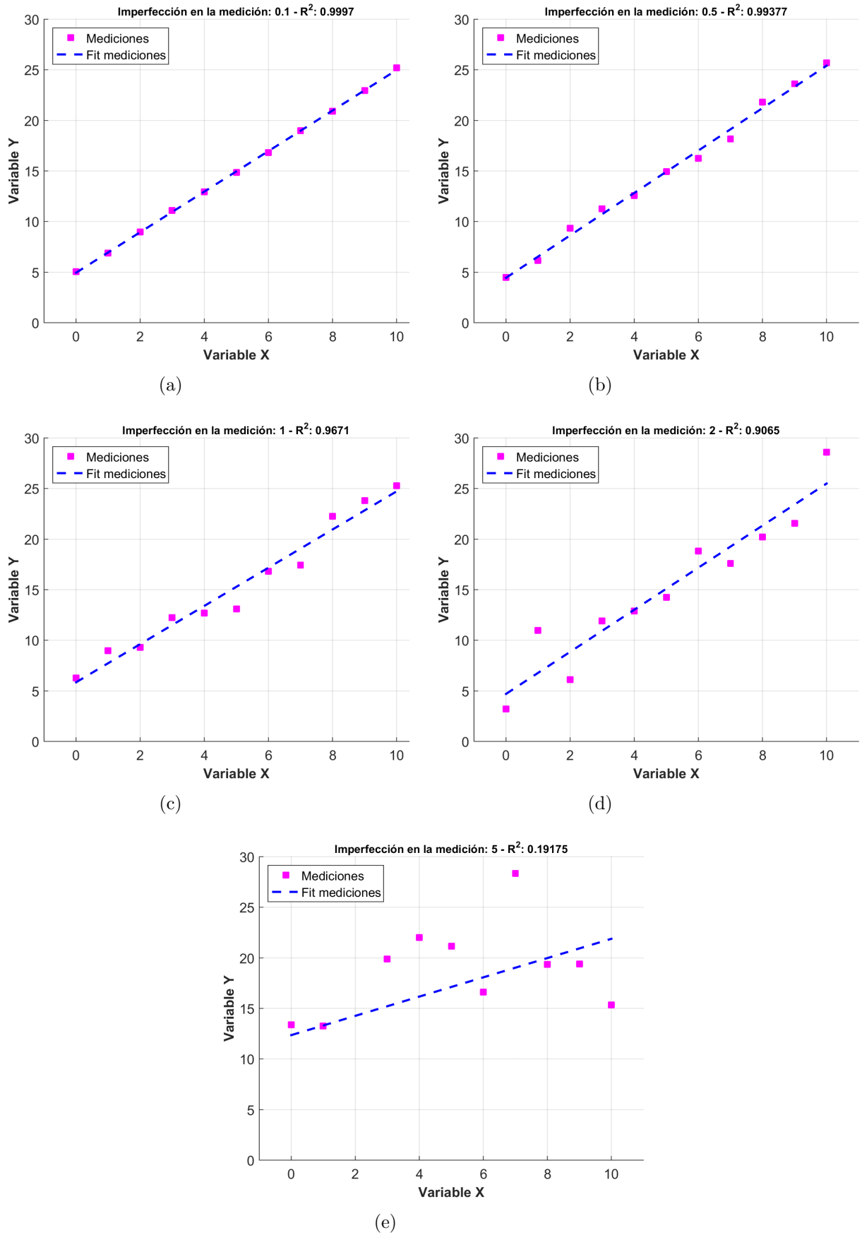
Figura 2: Ejemplos de aplicación del método de Mínimos Cuadrados a diferentes mediciones, utilizando un modelo lineal. (a) R^2=0,99970 , (b) R^2=0,99377 , (c) R^2=0,96710 , (d) R^2=0,90650 y (e) R^2=0,19175
