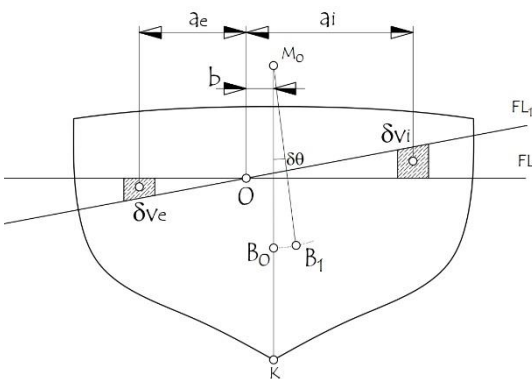
Fig. 6 - Determinación del radio metacéntrico
