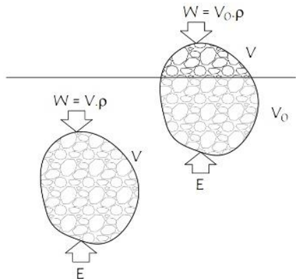
Fig. 1 - Empuje en cuerpo sumergido y flotador
