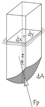
Fig. 2 - Fuerza actuante sobre un elemento de superficie de un flotador
