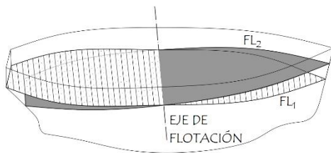
Fig. 4 – Flotaciones isocarenas
