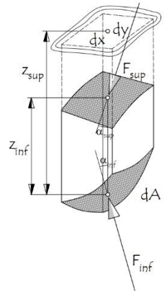
Fig. 3 - Fuerza actuante sobre un elemento de superficie de un cuerpo
