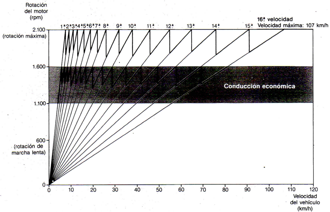
Gráfico Dientes de Sierra - LS 1630 Eje trasero: i=3,767:1
