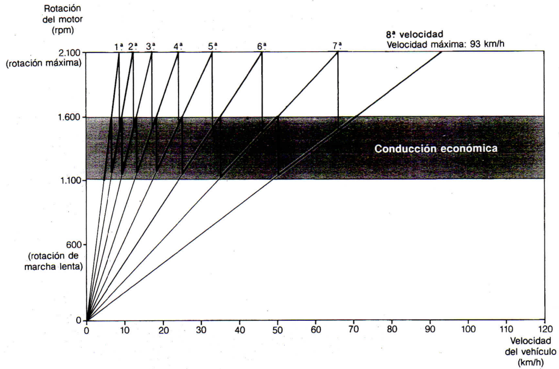
Gráfico Dientes de Sierra - L/LS 1625 Eje trasero: i=4,3:1
