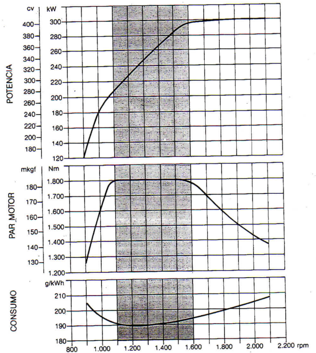
Curvas de Desempeño MB OM 447 LA - LS 1941
