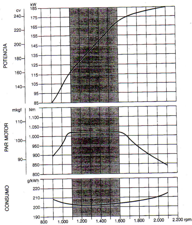
Curvas de Desempeño MB OM 449 A - L/LS 1625
