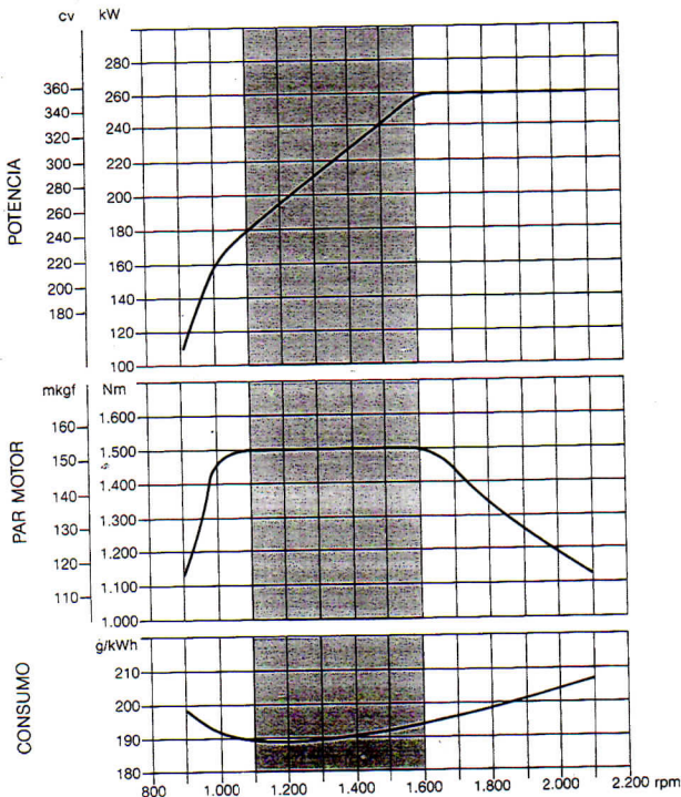
Curvas de Desempeño MB OM 447 LA - LS 1935
