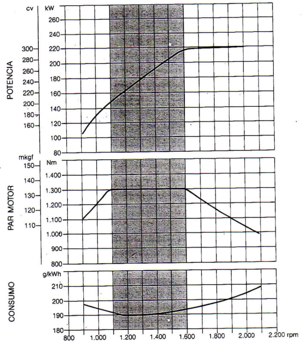
Curvas de Desempeño MB OM 449 LA - LS 1630
