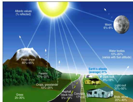
Fig. 1. El albedo 1
