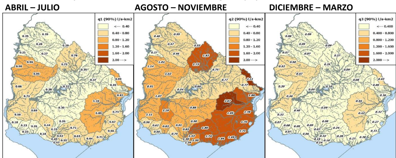
Figura 25 – Regionalización de caudales específicos estacionales q_j(90\%)
