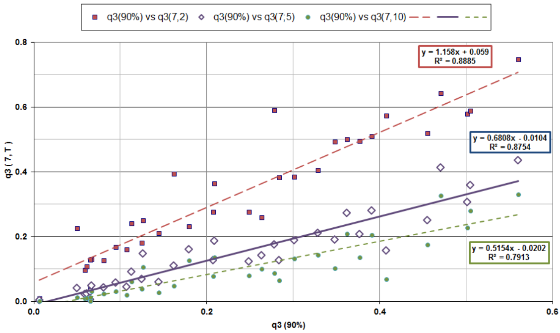
Figura IV-11.- Correlación entre q_3(7, T) y q_3(90\%) para distintos T (años)
