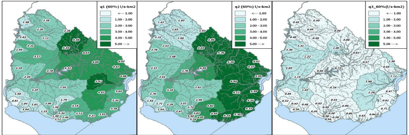
Figura 27 – Regionalización de caudales específicos estacionales q_j(60\%) Nivel 2 de codificación de subcuencas
