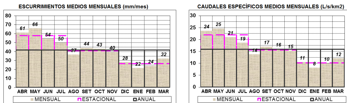
Figura 3 – Ciclos medios anuales de caudales – Vertiente del Río Uruguay (1980 – 2010) Estaciones hidrométricas del Servicio Hidrológico
