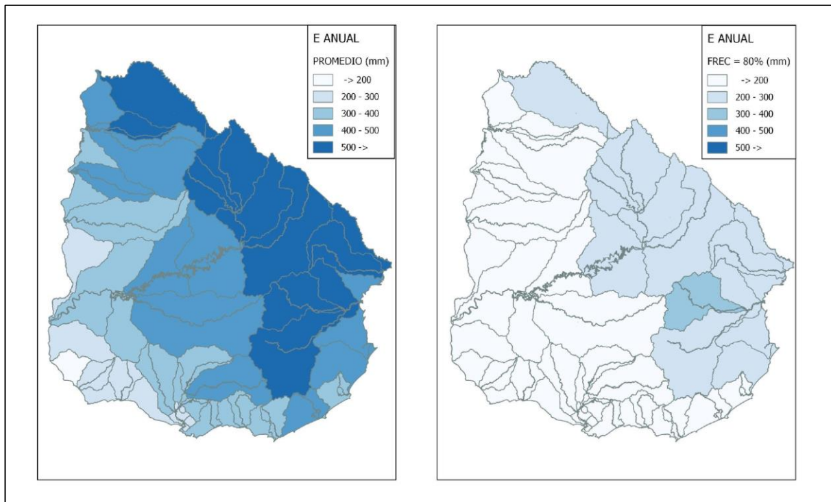
Figura 8 - Distribución geográfica de E_{med} y E_{(80\%)}
