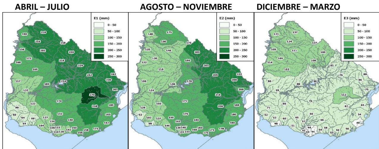
Figura 24 – Escurrimientos acumulados cuatrimestrales (mm)
