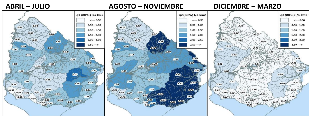
Figura 26 – Regionalización de caudales específicos estacionales q_j(80\%)
