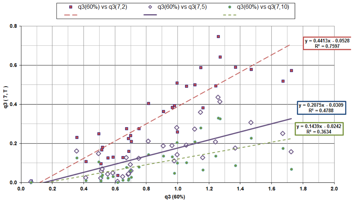
Figura IV-27.- Correlación entre q_3(7, T) y q_3(60\%) para distintos T (años)
