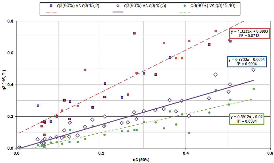
Figura IV-12.- Correlación entre q_3(15, T) y q_3(90\%) para distintos T (años)
