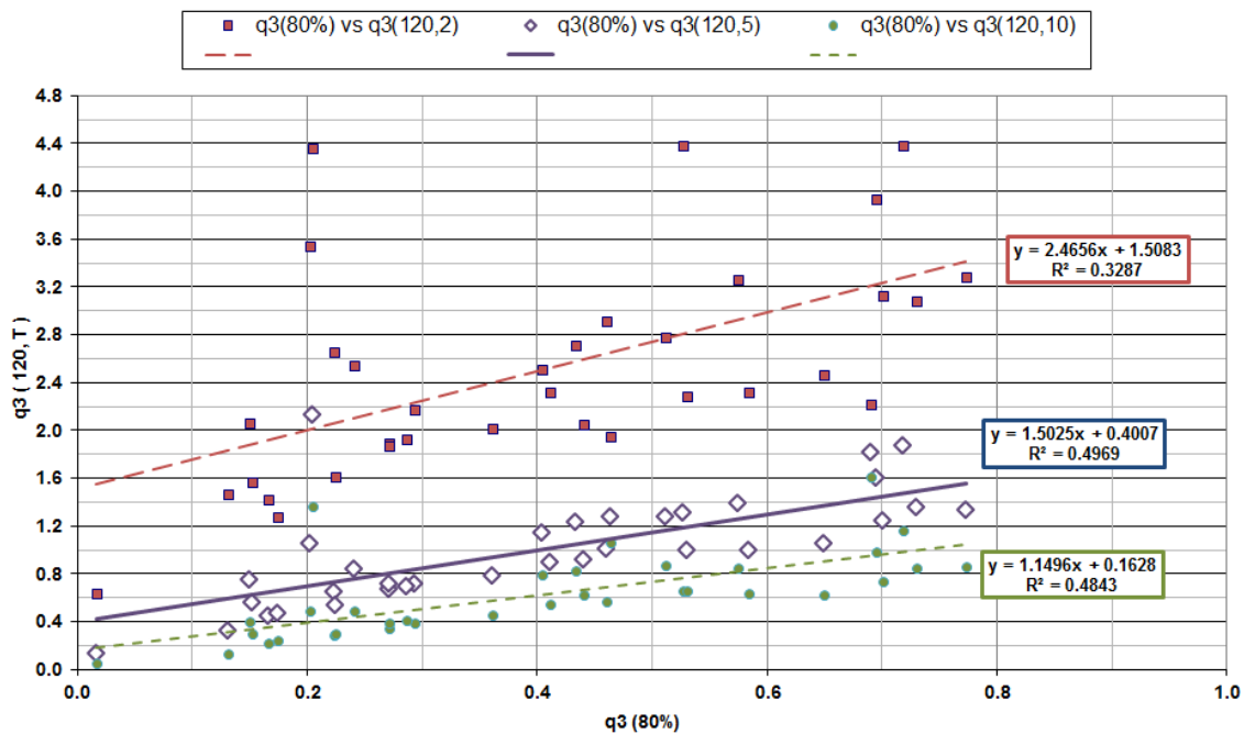
Figura IV-23.- Correlación entre q_3(120, T) y q_3(80\%) para distintos T (años)
