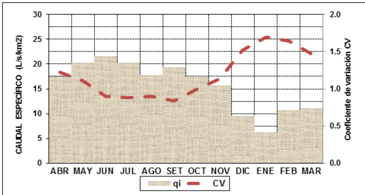
Figura 6 – Ciclo medio anual de caudales específicos q_i y coeficientes de variación CV (1980-2010) Estaciones hidrométricas del Servicio Hidrológico
