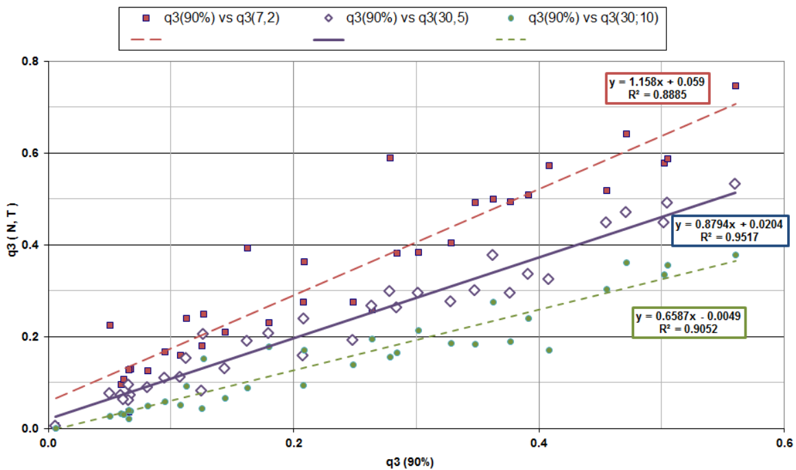
Figura 17 - Correlaciones q_3(N, T) vs q_3(90\%) (1980-2010)
