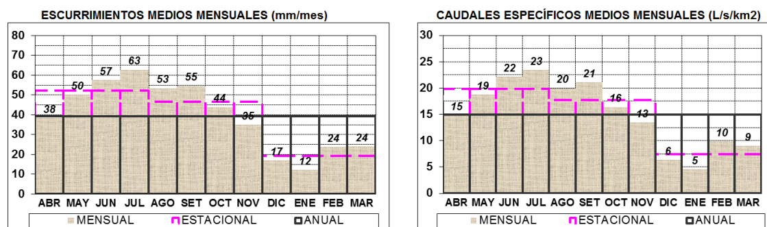
Figura 4 – Ciclos medios anuales de caudales – Vertiente Platense y Atlántica (1980 – 2010) Estaciones hidrométricas del Servicio Hidrológico
