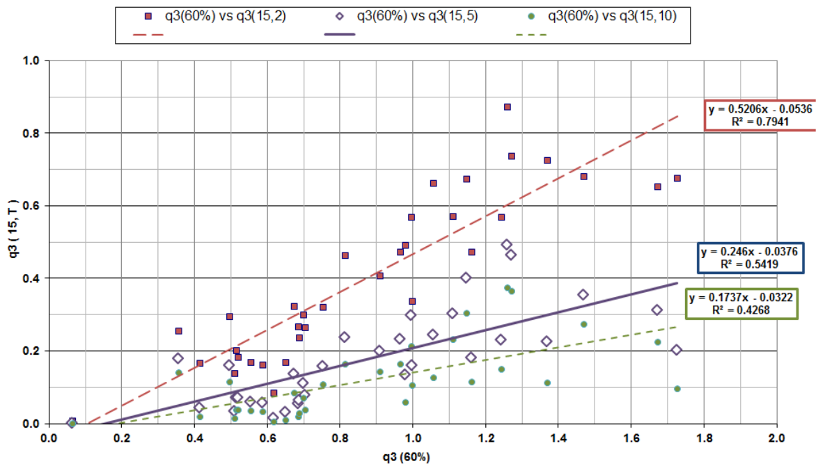
Figura IV-28.- Correlación entre q_3(15, T) y q_3(60\%) para distintos T (años)
