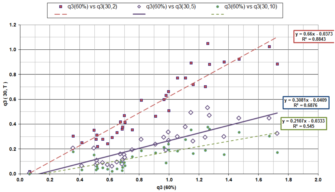
Figura IV-29.- Correlación entre q_3(30, T) y q_3(60\%) para distintos T (años)
