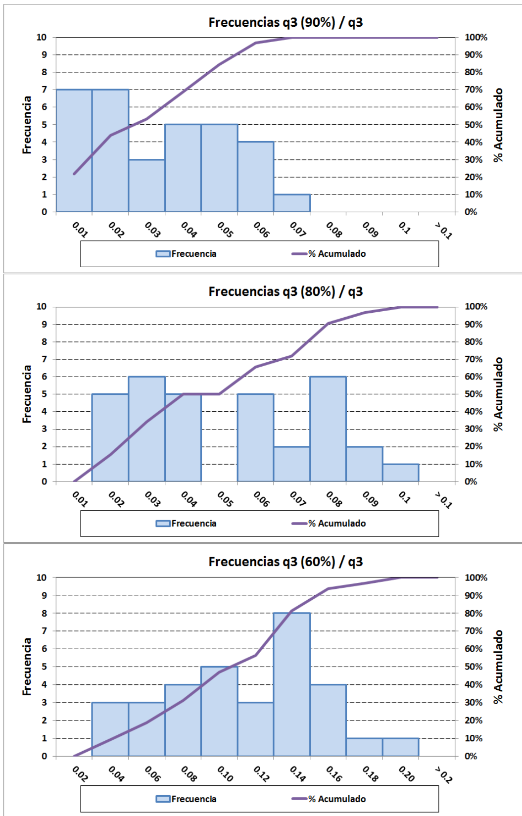
Figura 14 – Histogramas de q_3 (FF\%) / q_3 (1980-2010)
