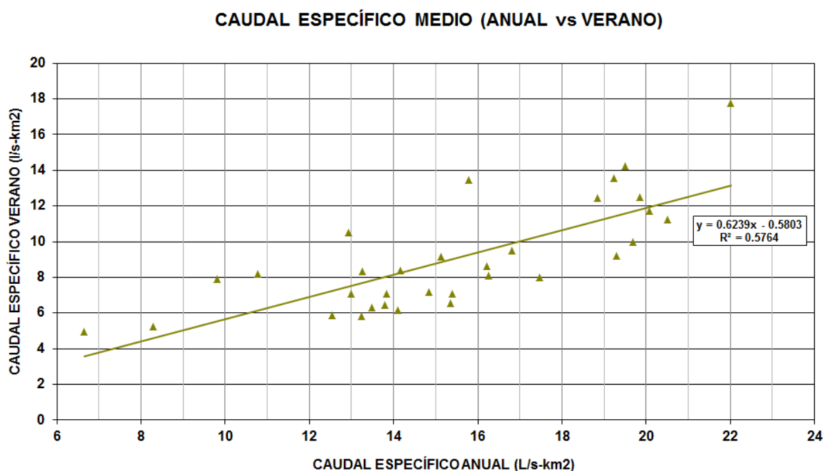
Figura 15 – Correlación q_3 vs q (1980-2010) Estaciones hidrométricas del Servicio Hidrológico
