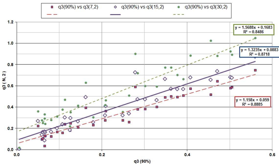
Figura IV-8.- Correlación entre q_3(N, 2) y q_3(90\%) para distintas duraciones N (días)
