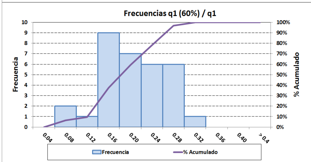
Figura 12 – Histogramas de q_1 (FF\%) / q_1 (1980-2010)
