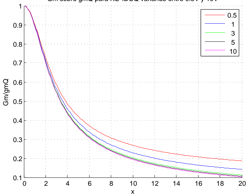
Gm sobre gmQ para RE*IDCQ variando entre 0.5V y 10V
