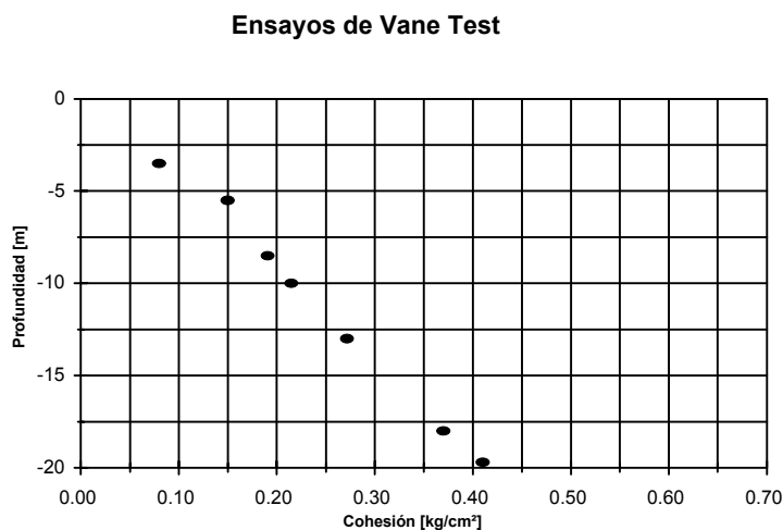
Figura N° 17: Resultados del ensayo de Vane test en un manto de arcilla blanda normalmente consolidada donde se midió una densidad efectiva \gamma' = 0,75 \text{ tn/m}^3
