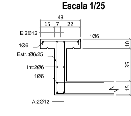
Sección V. 311-312-313 Escala 1/25
