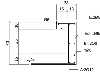
Sección V. 360 Escala 1/25
