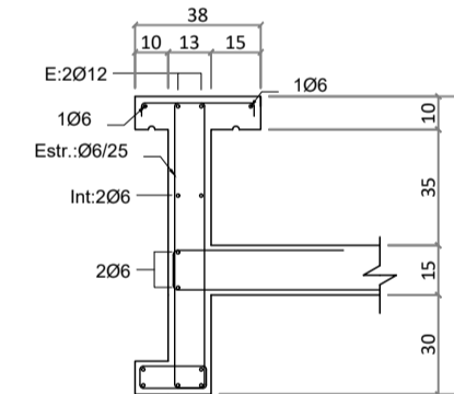
Sección V. 353-354 Escala 1/25
