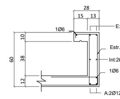
Sección V. 304 Escala 1/25
