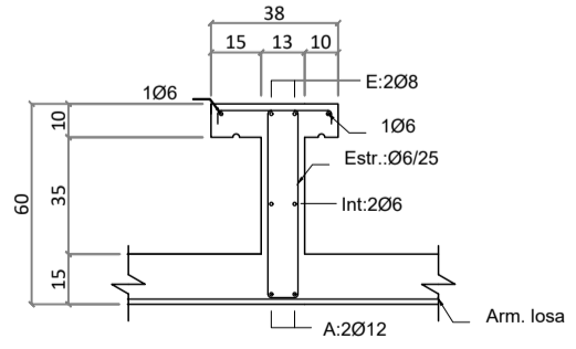
Sección V. 359 Escala 1/25
