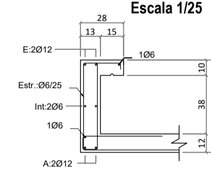
Sección V. 308 Escala 1/25
