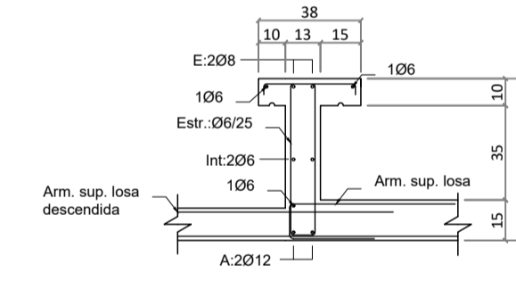
Sección V. 352 Escala 1/25
