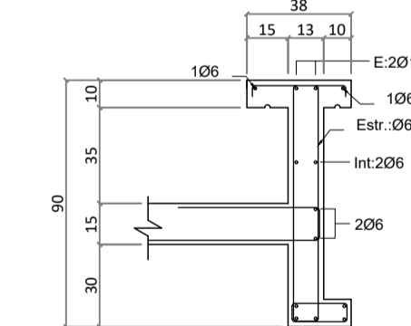
Sección V. 357-358 Escala 1/25
