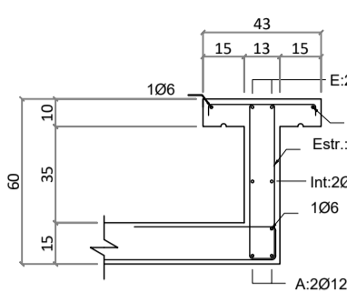
Sección V. 301-302-303 Escala 1/25
