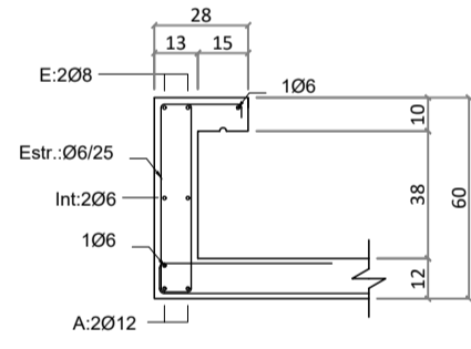
Sección V. 351 Escala 1/25
