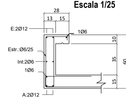
Sección V. 305-306 Escala 1/25
