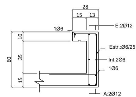
Sección V. 307 Escala 1/25
