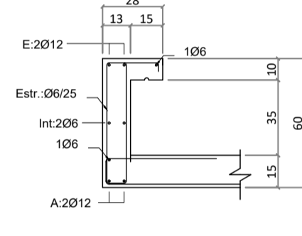
Sección V. 310 Escala 1/25
