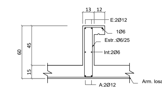
Sección V. 356 Escala 1/25
