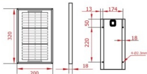
DIMENSIONES/ DIMENSIONS ESF-5MA ESF-5PA
