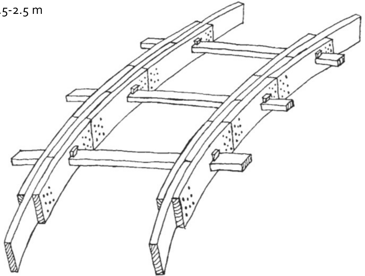
Fig. 3 - ARRIOSTRAMIENTO LATERAL. ARMADURA TIPO DE L'ORME
