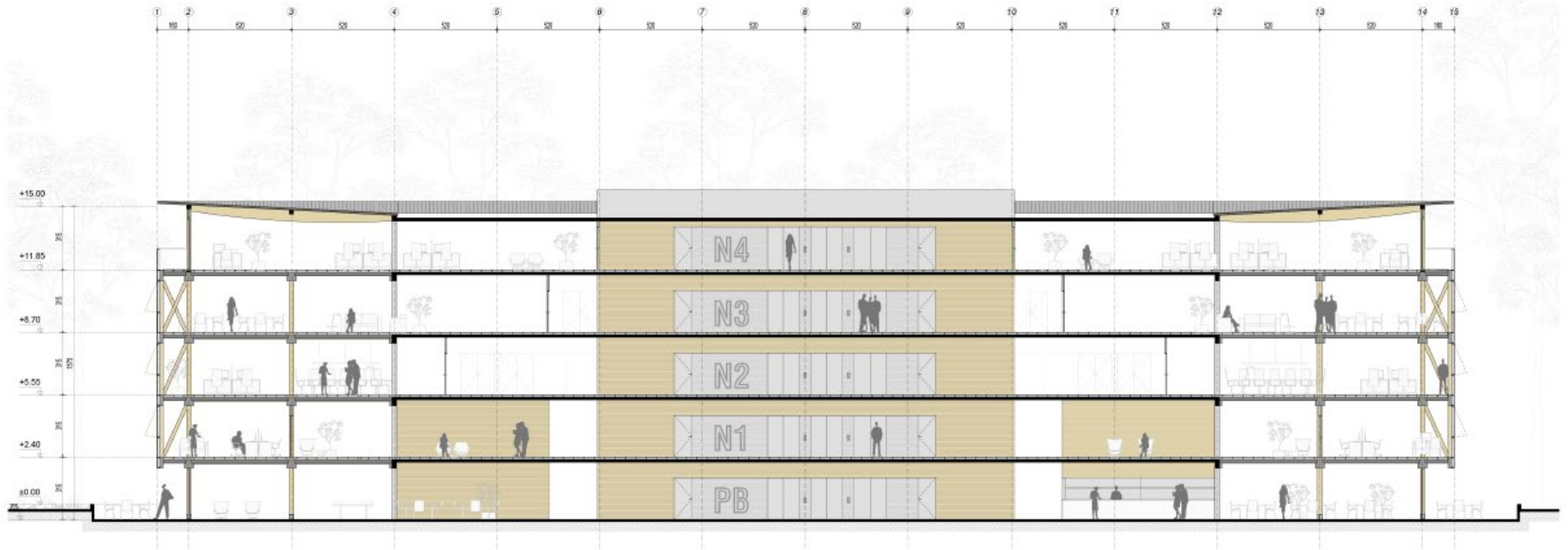
Corte longitudinal
