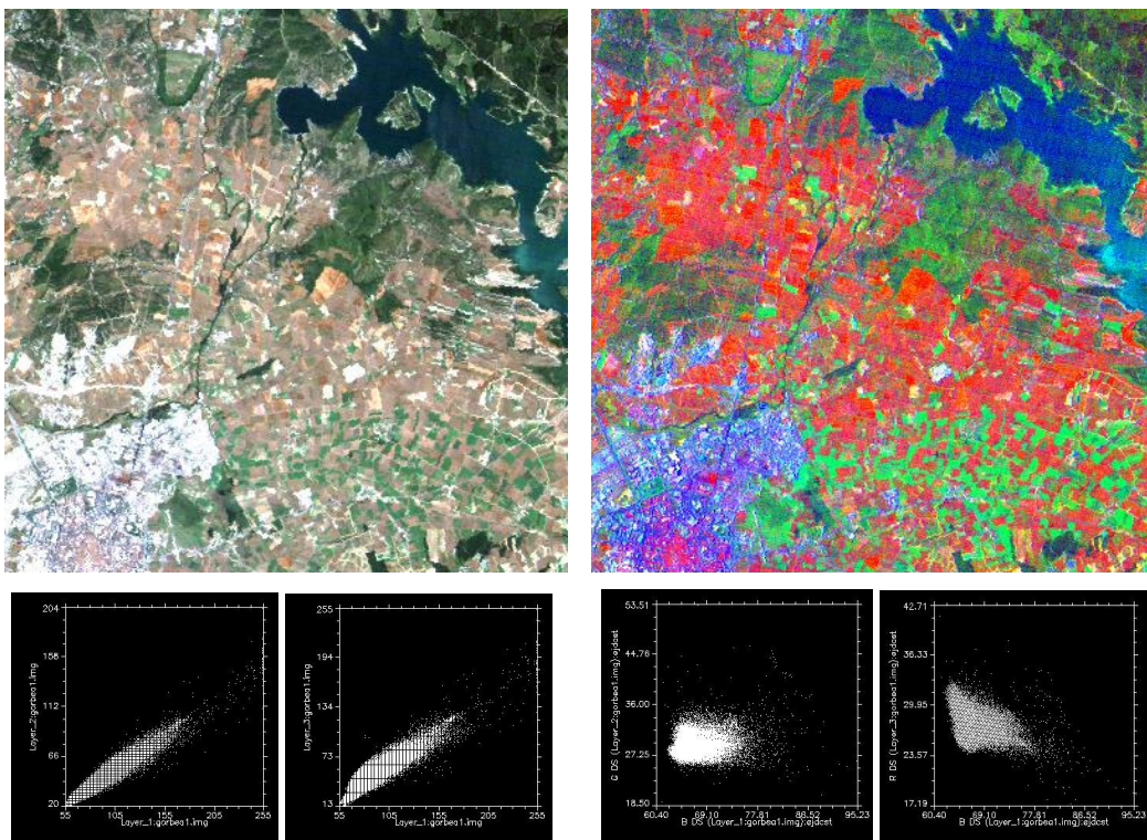
Figura 4.- Ejemplo de aplicación del realce espectral por decorrelación. La imagen de la izquierda representa una combinación en color natural con elevado contraste pero con una gran correlación entre bandas, como puede apreciarse en sus dos diagramas de dispersión (relacionan las bandas rojo/verde y rojo/azul). El resultado de la decorrelación se muestra en la imagen de la derecha,
