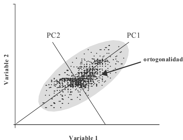
Figura 1.- Diagrama de dispersión de dos variables y direcciones de los componentes principales resultantes (PC1 y PC2).
