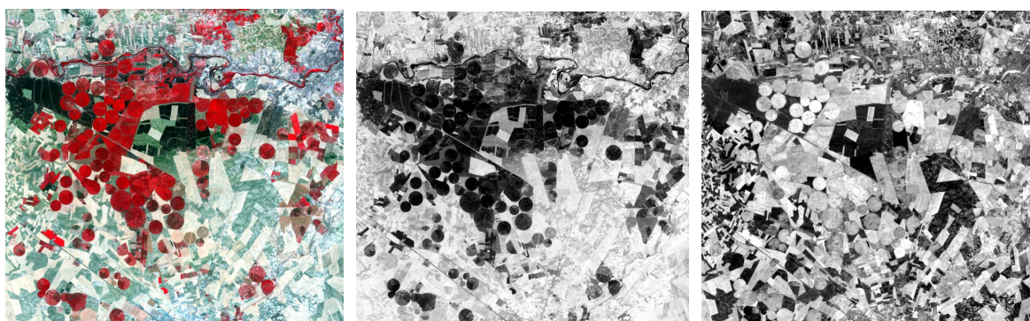
Figura 2.- Combinación en falso color infrarrojo (bandas 432-RGB) de la imagen Landsat-TM de los regadíos del río Júcar (izquierda). Imágenes de los componentes principales 1º y 2º (centro y derecha) de la imagen de las 7 bandas espectrales original.
