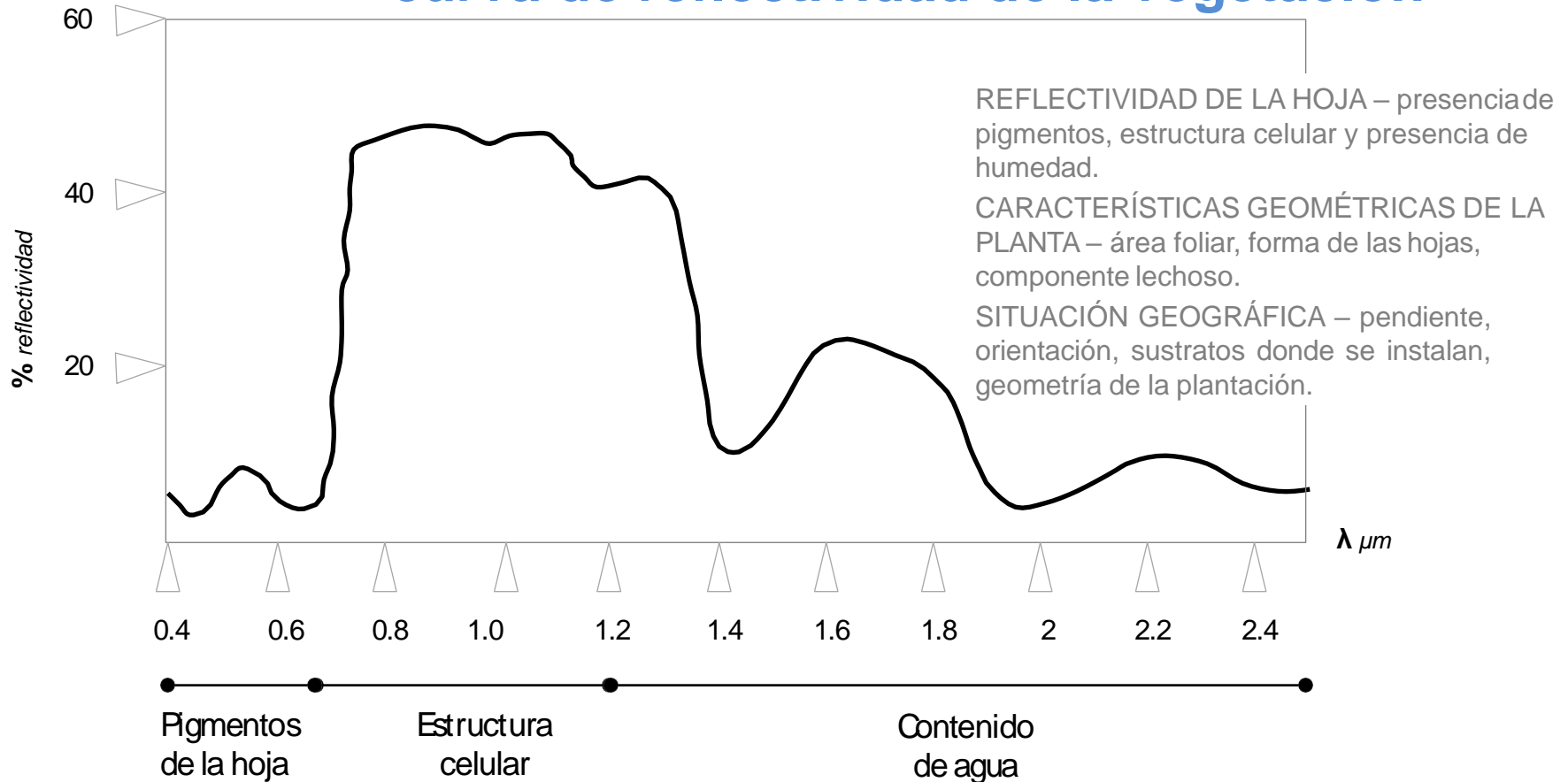
Figura – curvas de reflectividad - Emilio Chuvieco
