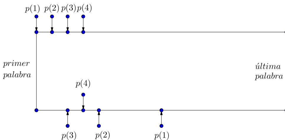
Figura 1: Iteraciones para encontrar la cuarta palabra en un diccionario de 17 palabras
