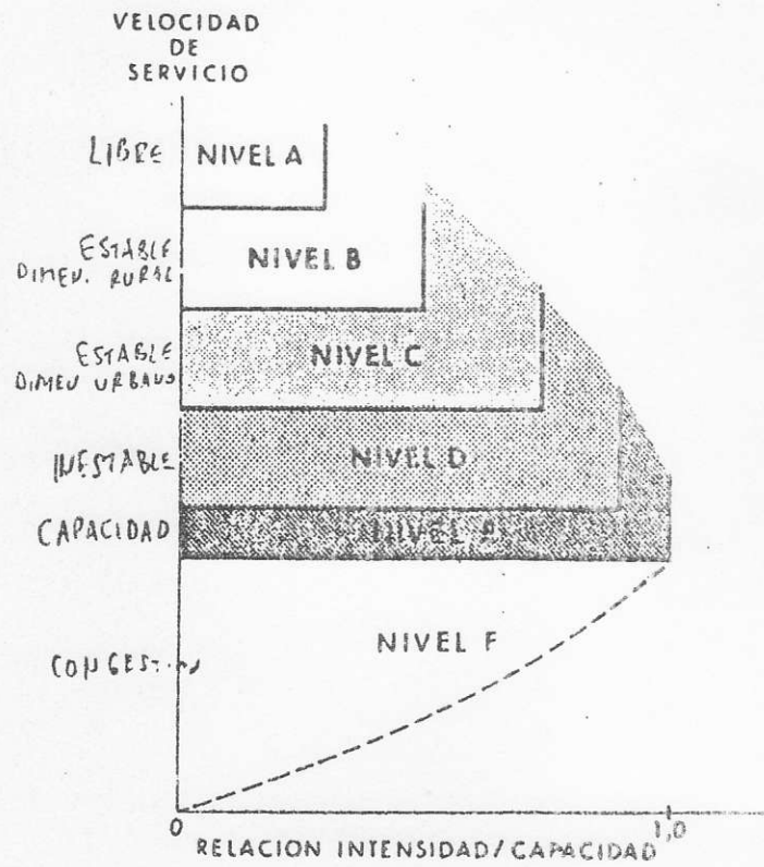
DEFINICION DE NIVELES DE SERVICIO EN CIRCULACION CONTINUA.
