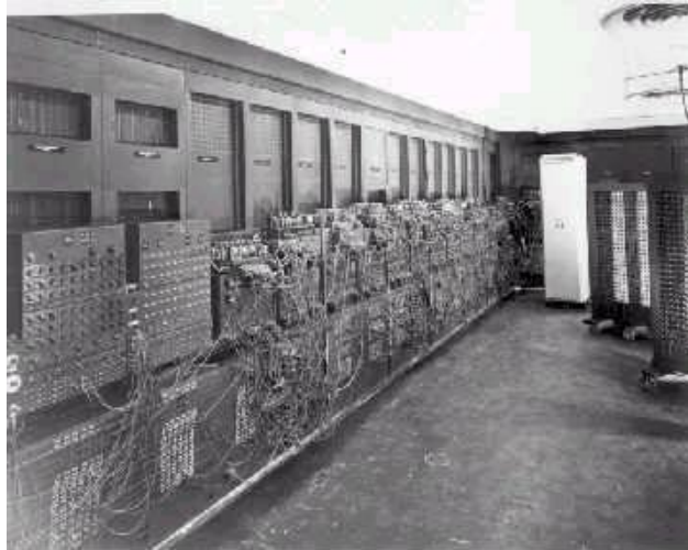
ENIAC
