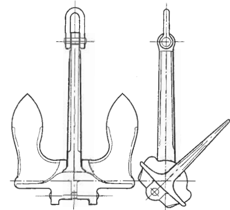
Baldt anchor
