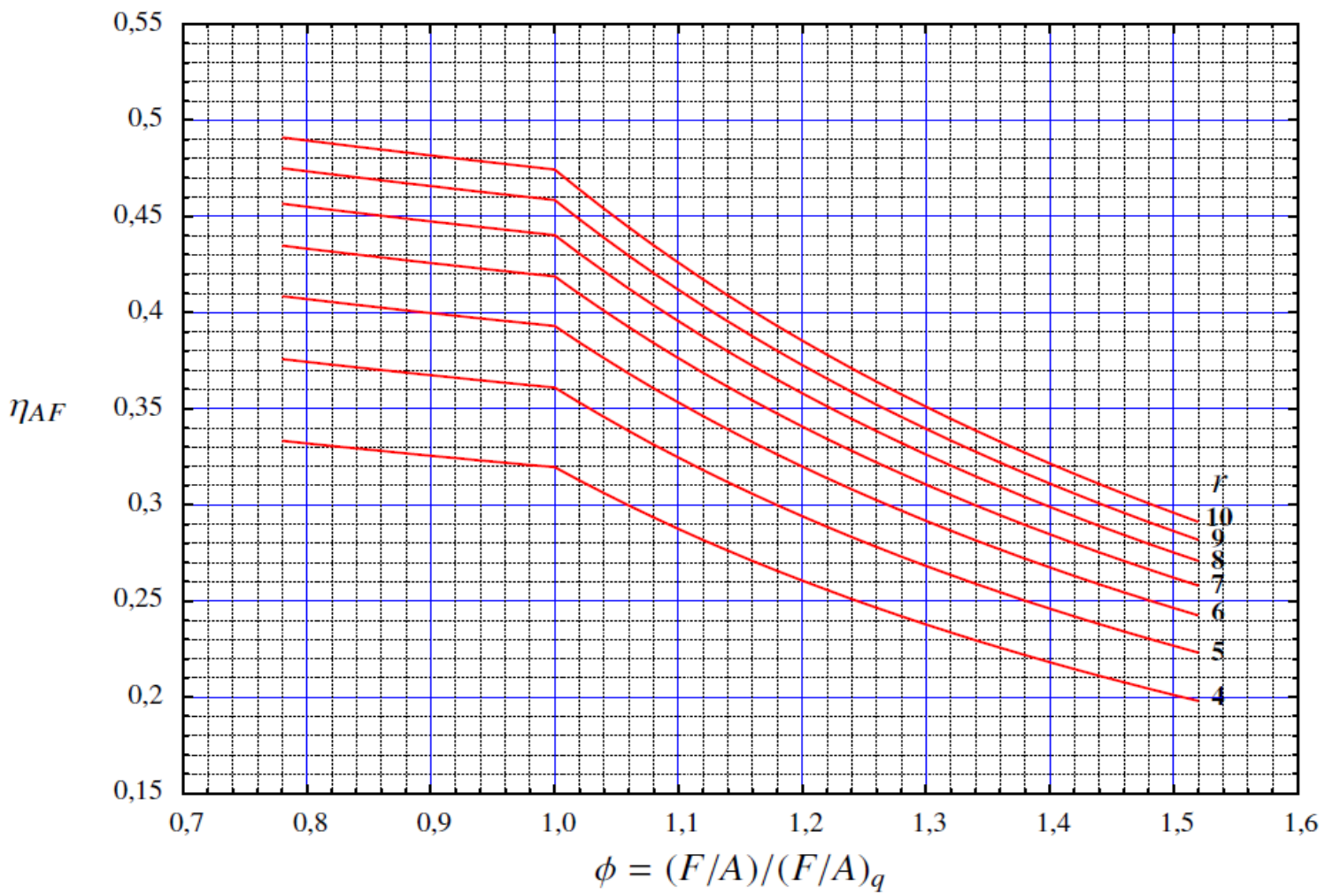
Figure 1: Rendimientos calculados a partir de la resolución del ciclo teórico sin considerar gases residuales, tomando como datos iniciales p_{in} = p_{ex} = 1\text{atm} y T_{in} = 289.15\text{K}
