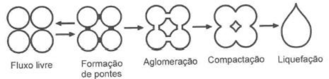
Figura 2. Alterações durante o processo de caking .
