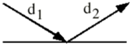
Reflexión
