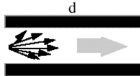
Onda guiada
