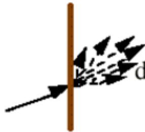
Absorción
