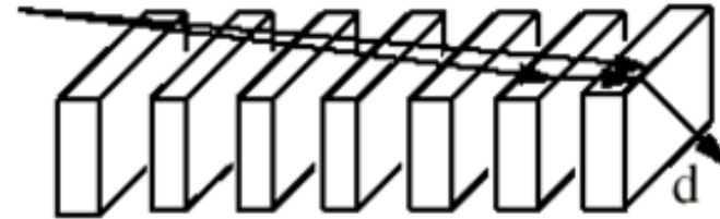
Difracción Múltiple
