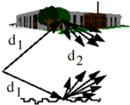
Difusión
