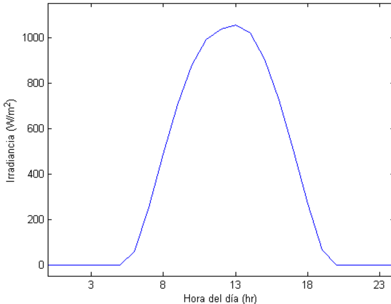
Irradiancia horaria típica en plano horizontal (verano)
