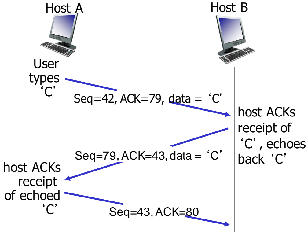
simple telnet scenario
