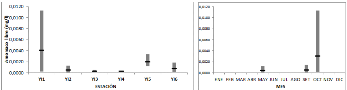
Figura 47: Variación espacial (izquierda) y temporal (derecha) del Amoníaco libre con sus máximos, mínimos y promedios en el río Yí durante 2019.
