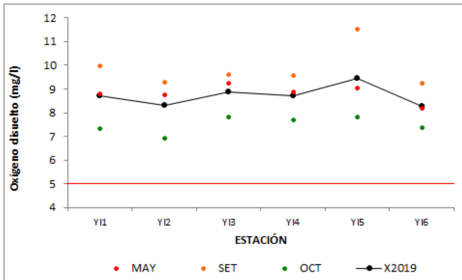
Figura 13: Fluctuaciones del oxígeno disuelto a lo largo del río Yí.
