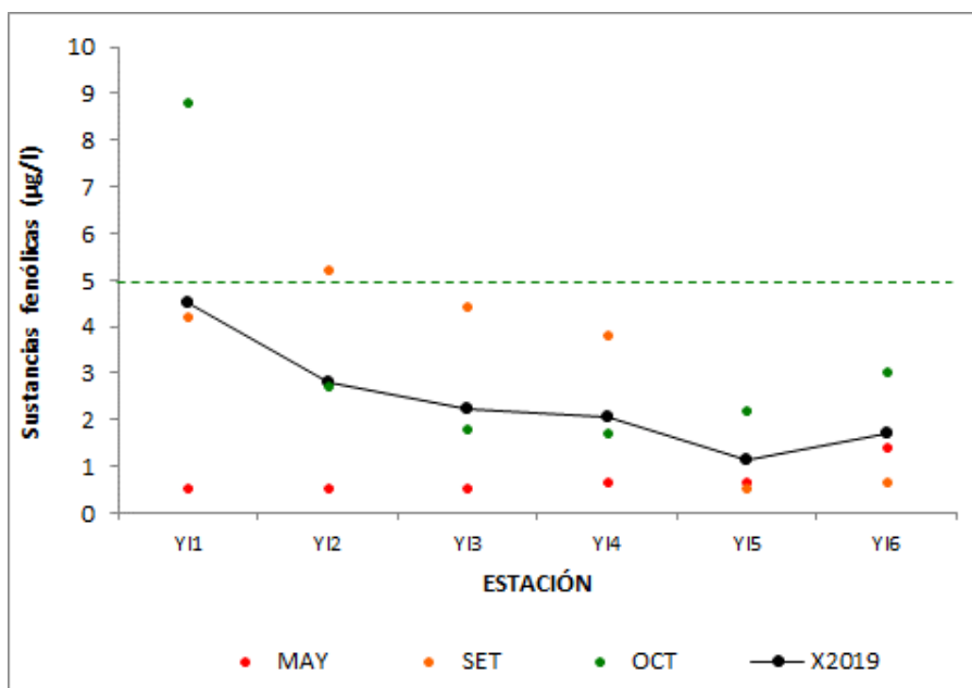
Figura 26: Fluctuaciones de las sustancias fenólicas a lo largo del río Yí.
