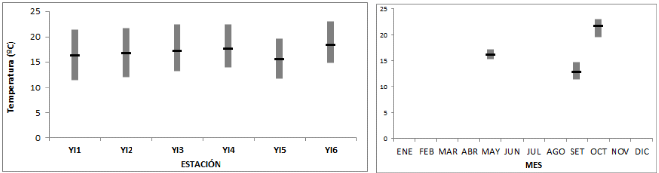
Figura 8: Variación espacial (izquierda) y temporal (derecha) con sus máximos, mínimos y promedios de la temperatura en el Río Yí durante 2019.
