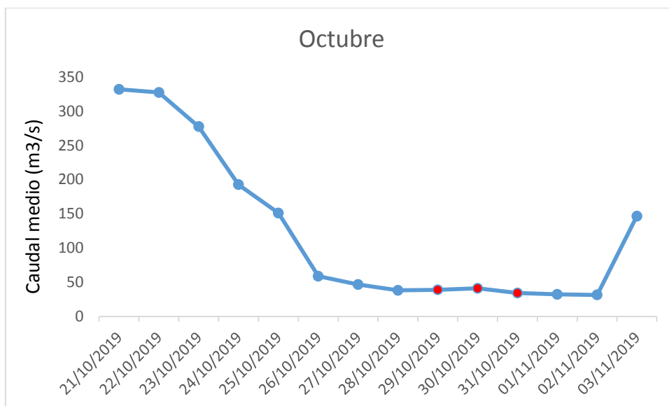
Figura 6: Caudal diario en el aforo de la ciudad de Durazno en la campaña de monitoreo del mes de Octubre y en la semana previa. En rojo se muestran los caudales correspondientes a los días de monitoreo.
