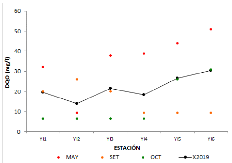
Figura 19: Fluctuaciones de la Demanda Química de oxígeno a lo largo del río Yí.
