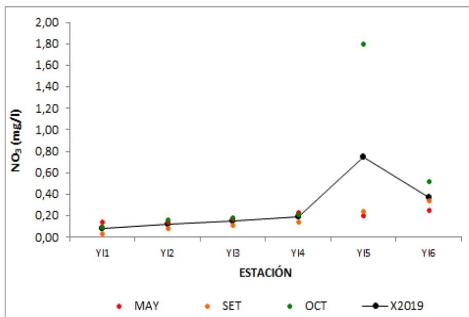
Figura 38: Fluctuaciones del Nitrato a lo largo del río Yí.
