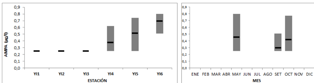
Figura 57: Variación espacial (izquierda) y temporal (derecha) de la concentración de AMPA en el río Yí durante 2019.
