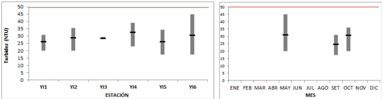
Figura 16: Variación espacial (izquierda) y temporal (derecha) de la turbidez con sus máximos, mínimos y promedios en el río Yí durante 2019. ---.La línea roja continua marca el estándar de 50 NTU fijado en el Decreto 253/79.
