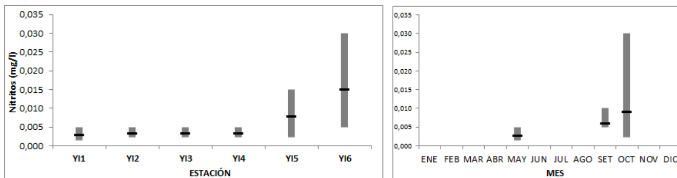
Figura 41: Variación espacial (izquierda) y temporal (derecha) de los Nitritos, con sus máximos, mínimos y promedios en el río Yí durante 2019.
