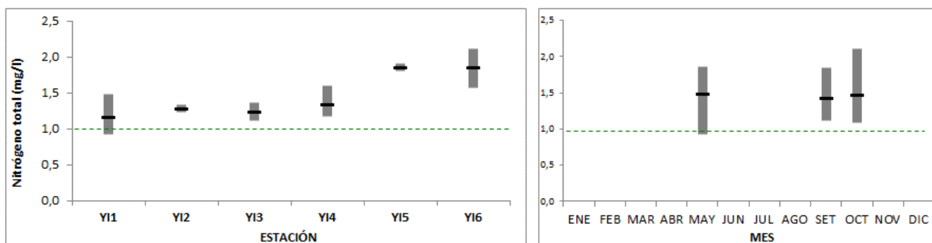
Figura 43: Variación espacial (izquierda) y temporal (derecha) del Nitrógeno Total, con sus máximos, mínimos y promedios en el río Yí durante 2019. ---.La línea verde punteada marca el límite de 1mg/L propuesto por la Mesa Técnica del Agua en 2017.
