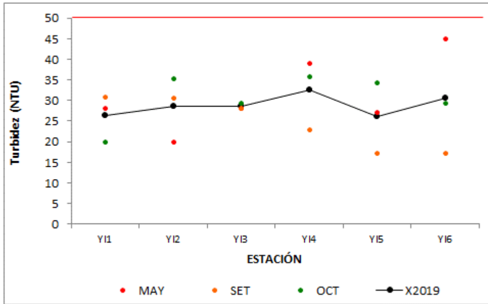
Figura 15: Fluctuaciones de la turbidez lo largo del río Yí.
