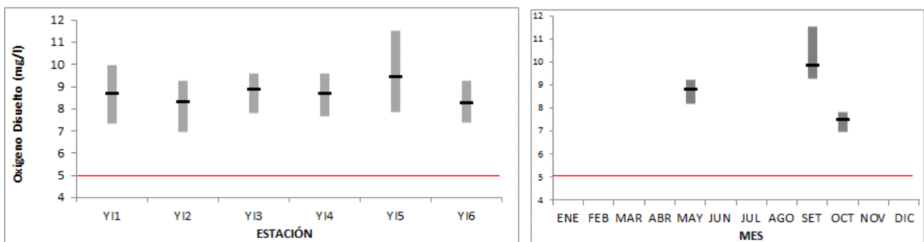
Figura 14: Variación espacial (izquierda) y temporal (derecha) del oxígeno disuelto, con sus máximos, mínimos y promedios en el río Yí durante 2019. ---.La línea roja continua marca el estándar de 5 mg/L fijado en el Decreto 253/79.
