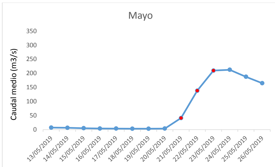
Figura 4: Caudal diario en el aforo de la ciudad de Durazno en la campaña de monitoreo del mes de mayo y en la semana previa. En rojo se muestran los caudales correspondientes a los días de monitoreo.
