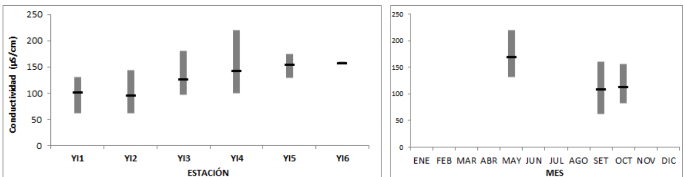
Figura 10: Variación espacial (izquierda) y temporal (derecha) con sus máximos, mínimos y promedios de la conductividad en el Río Yí durante 2019.
