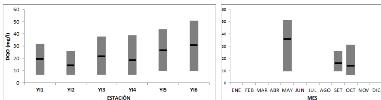
Figura 20: Variación espacial (izquierda) y temporal (derecha) de la Demanda Química de Oxígeno en el río Yí durante 2019.
