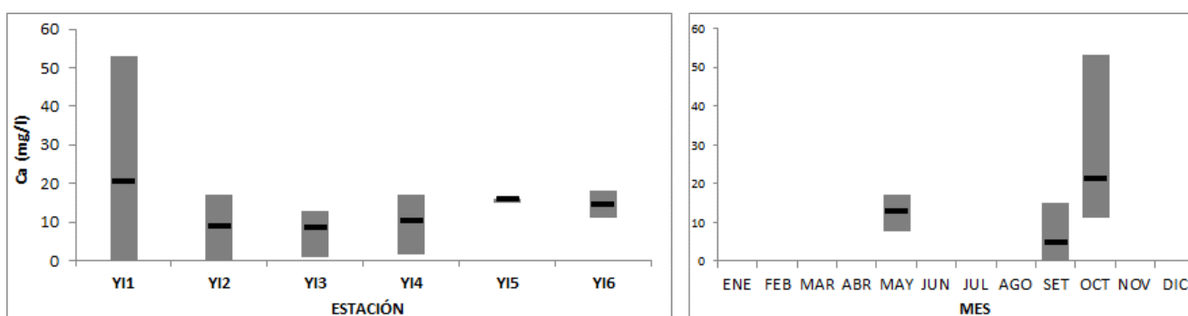
Figura 29: Variación espacial (izquierda) y temporal (derecha) de la concentración de Calcio, con sus máximos, mínimos y promedios en el río Yí durante 2019.
