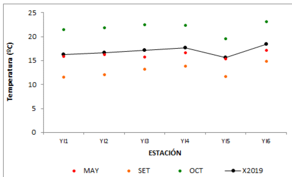
Figura 7: Fluctuaciones de la temperatura lo largo del Río Yí.
