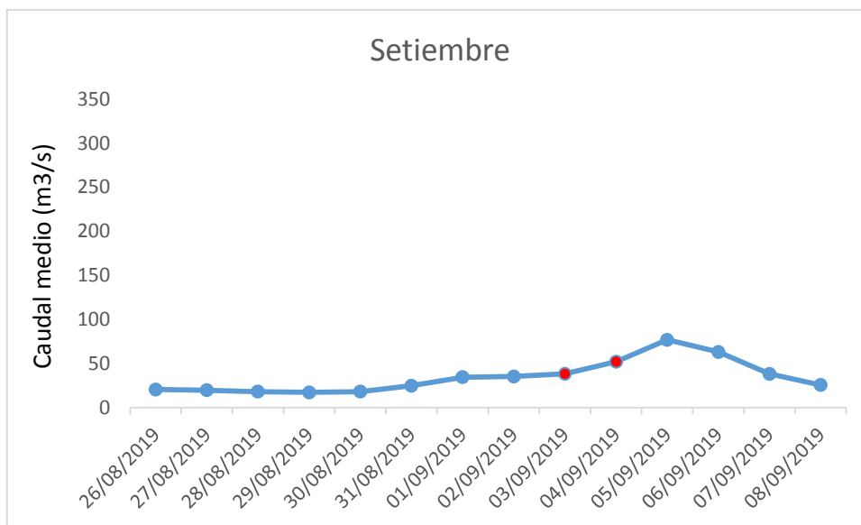
Figura 5: Caudal diario en el aforo de la ciudad de Durazno en la campaña de monitoreo del mes de setiembre y en la semana previa. En rojo se muestran los caudales correspondientes a los días de monitoreo.
