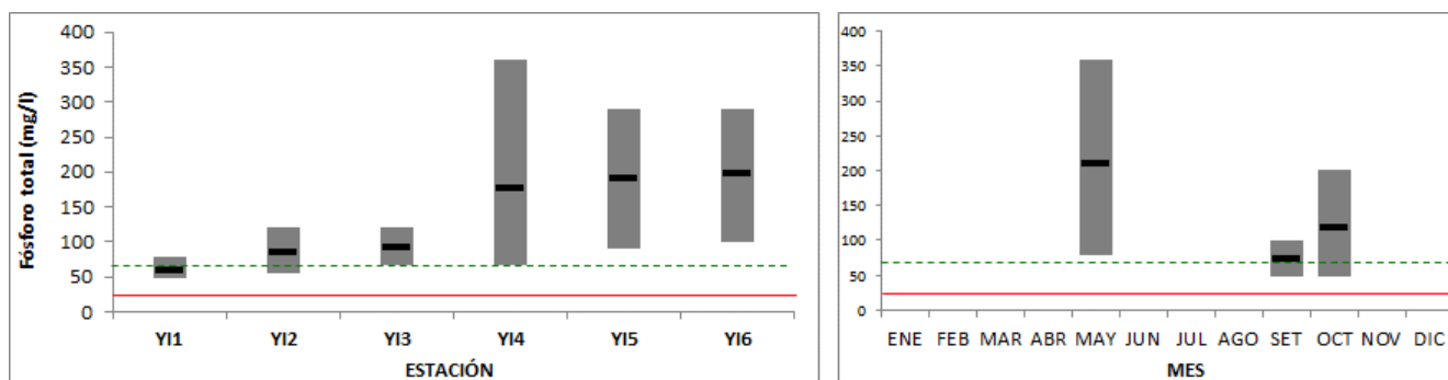
Figura 51: Variación espacial (izquierda) y temporal (derecha) del Fósforo Total con sus máximos, mínimos y promedios en el río Yí durante 2019.
