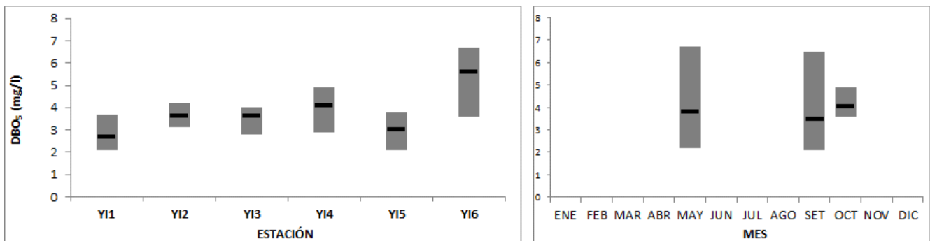
Figura 18: Variación espacial (izquierda) y temporal (derecha) de la demanda biológica de oxígeno, con sus máximos, mínimos y promedios en el río Yí durante 2019.
