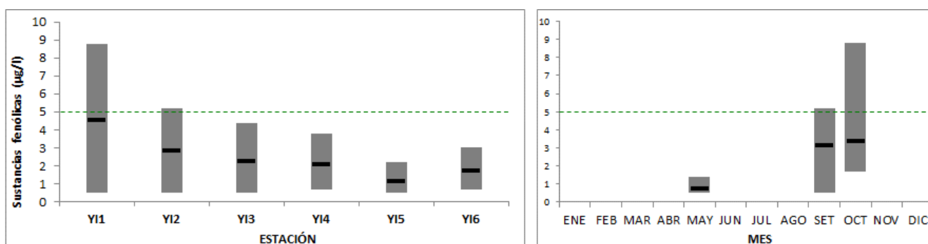
Figura 27: Variación espacial (izquierda) y temporal (derecha) de las sustancias fenólicas con sus máximos, mínimos y promedios en el río Yí durante 2019. ---.La línea verde punteada marca el límite máximo de 5 µg/L sugerido por GESTA agua en 2014.
