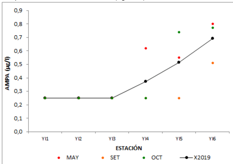
Figura 56: Fluctuaciones de la concentración de AMPA a lo largo del río Yí
