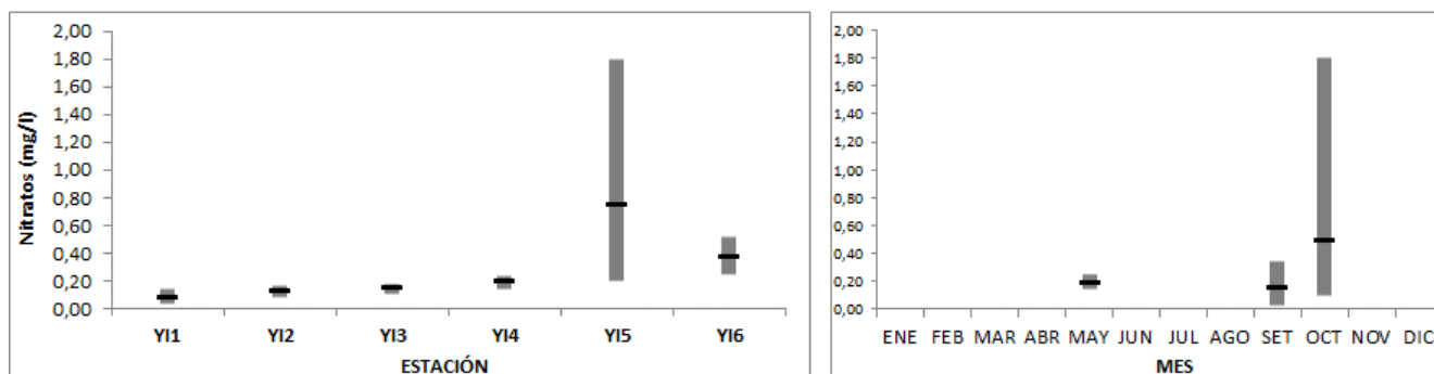
Figura 39: Variación espacial (izquierda) y temporal (derecha) del Nitrato, con sus máximos, mínimos y promedios en el río Yí durante 2019.
