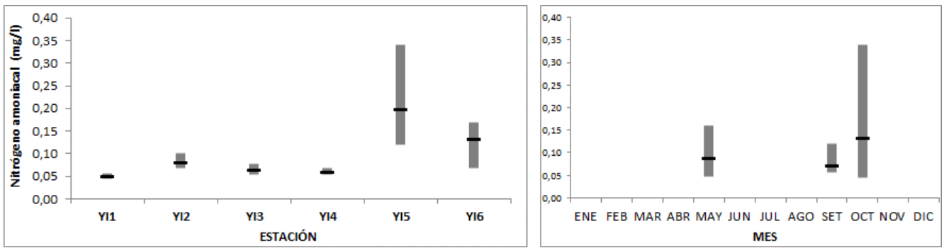
Figura 45: Variación espacial (izquierda) y temporal (derecha) del Nitrógeno amoniacal con sus máximos, mínimos y promedios en el río Yí durante 2019.
