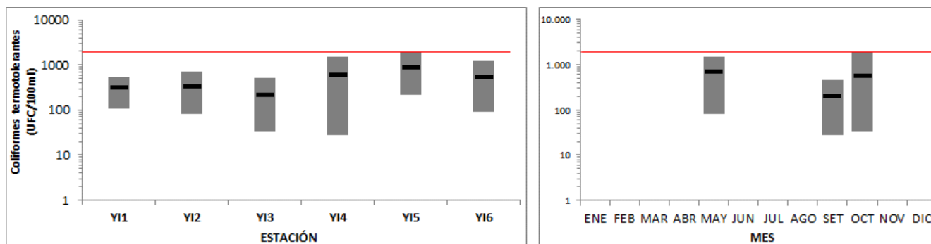
Figura 53: Variación espacial (izquierda) y temporal (derecha) de la concentración de Coliformes termotolerantes con sus máximos, mínimos y promedios en el río Yí durante 2019.
