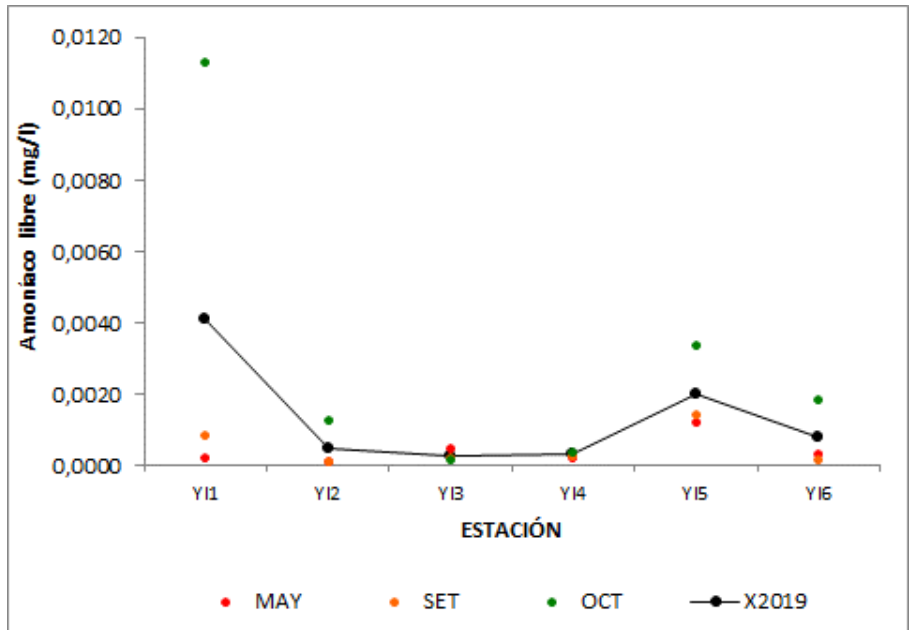
Figura 46: Fluctuaciones del Amoníaco libre a lo largo del río Yí
